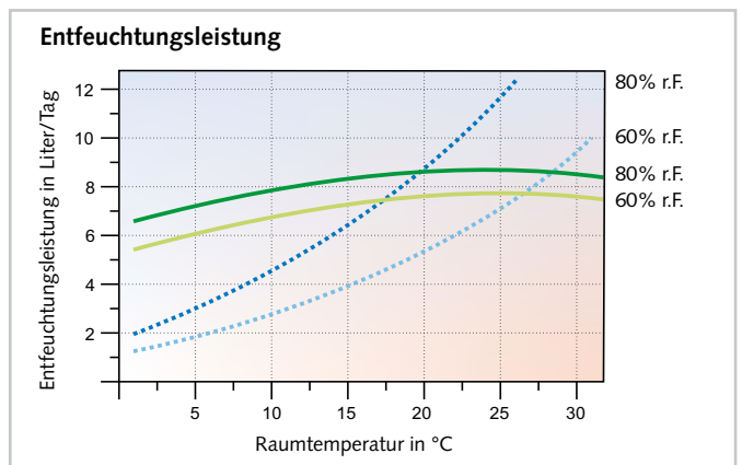
— REMKO ASF 100 mit Adsorptions-Rotor
